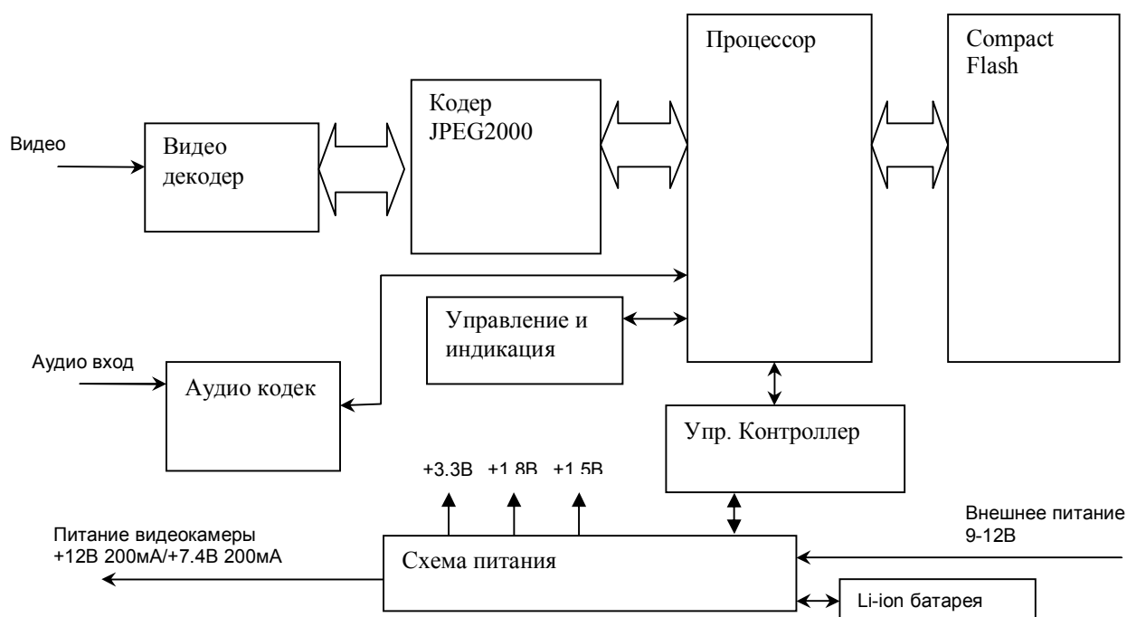
Рисунок 1.2 . Функциональная блок-схема видеонакопителя «МВН-01»
