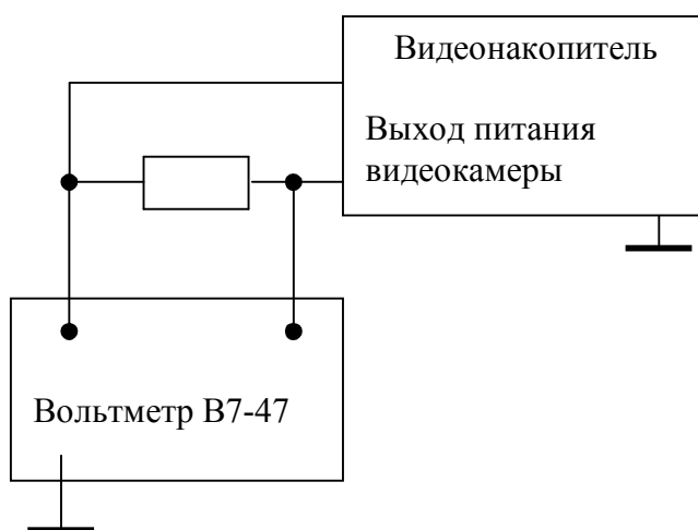
Рисунок 3.1 Схема рабочего места для проверки питания видеокамеры ( R = 62 \text{ Ома} для 12 В и 33 Ома для 6В)
